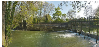
Barrage et vanne. Phot. Thierry Kuntz IVR26_20112102812NUC4A
