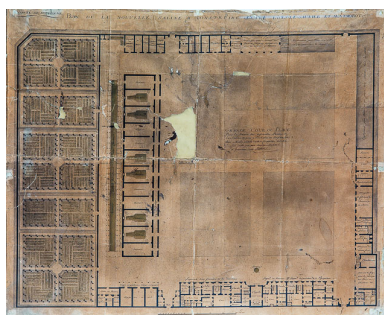
Plan de la nouvelle saline à construire entre Lons-le-Saunier et Montmorot. Phot. Jérôme Mongreville IVR43_19943900505XA
