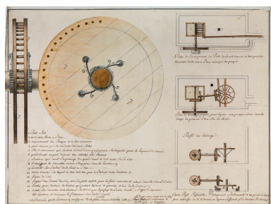
[Projet de déplacement de la roue hydraulique du Puits Salé et de nouveau système moteur combiné avec un manège à cheval].
