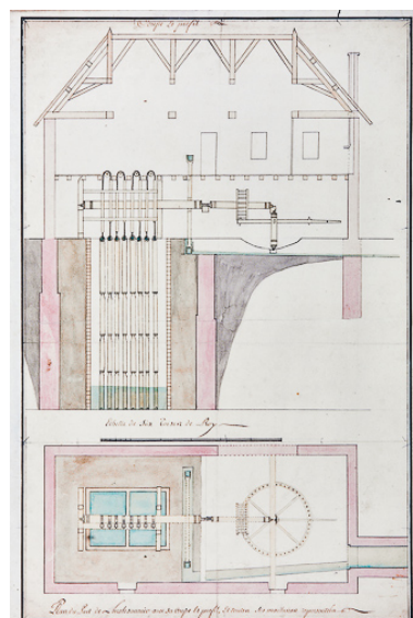
Plan du Puit de Lons le Saulnier avec sa coupe et profil, et toutes ses machines représentées. Phot. Jérôme Mongreville, Autr. Meynier IVR43_19943900468XA
