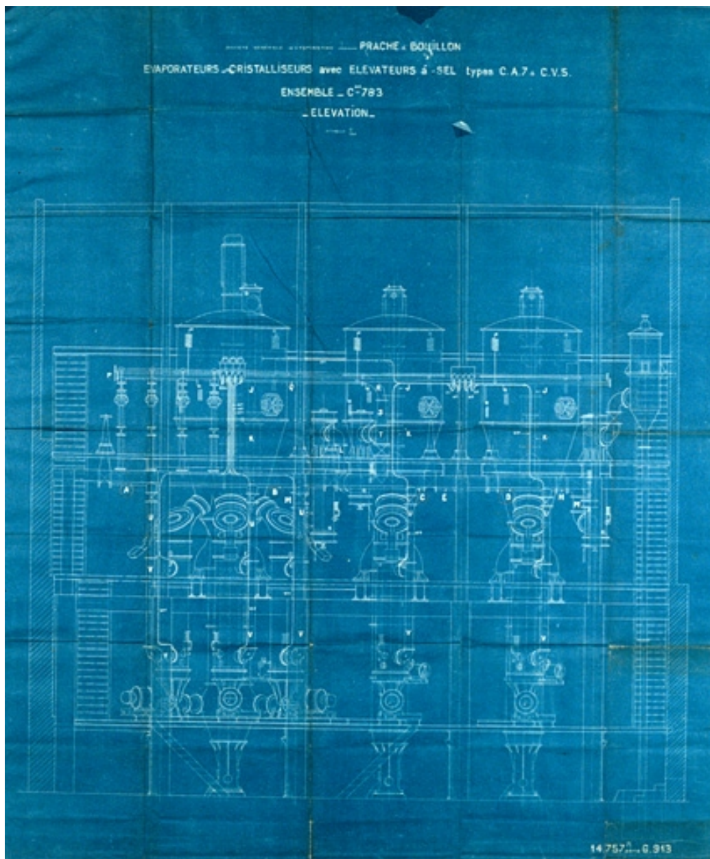
Evaporateurs-Cristalliseurs avec élévateurs à sel types C.A.7 & C.V.5. Ensemble - Cde 783. Elévation.
