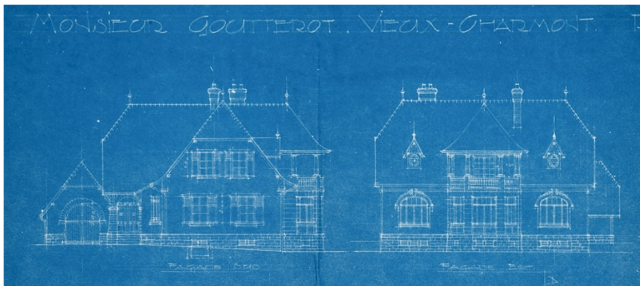
M. Goutterot. Projet d'habitation. Façades sud et est. Elévations, tirage à l'ammoniac, dressé par l'architecte soussigné [Reess], échelle 1/100, 23 mars 1929.
