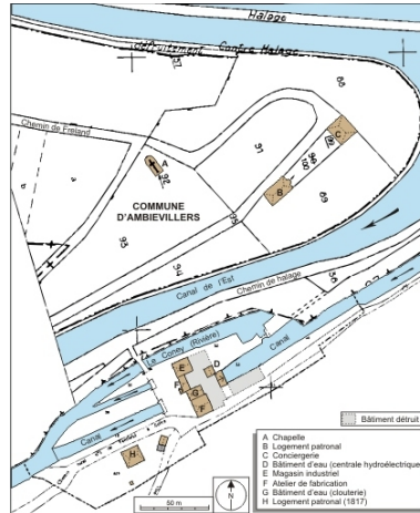
Plan-masse et de situation. Montage d'extraits de plans cadastraux numérisés, 2008, section A, 1:1250 et Ambiéville, section AD, 1: 2000, le tout réduit à 1:1700. Source : Direction générale des Finances Publiques - Cadastre ; mise à jour : 2008. Dess. André Céréza IVR43_20087000188NUCA
