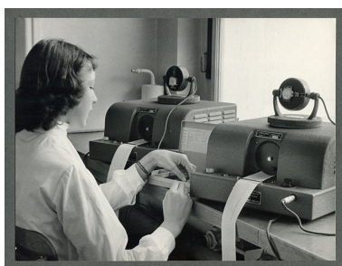
Ouvrière au travail : contrôle de marche au chronocomparateur (Vibrograf Lepaute), années 1960. IVR43_20182500797NUC4A
