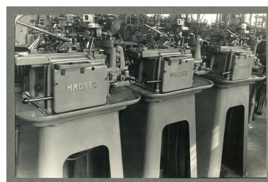
Machines de la société Hauser, années 1960. IVR43_20182500789NUC4A
