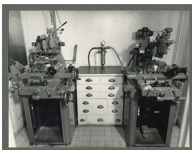
Atelier de métrologie : machines à contrôler, années 1960. IVR43_20182500785NUC4A
