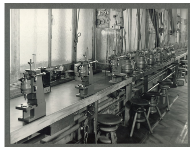
Perceuses d'établi, années 1960. IVR43_20182500780NUC4A
