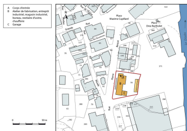
Plan-masse et de situation. Dess. Mathias Papigny IVR43_20162501494NUDA
