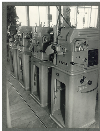
Machines à fraiser (contourneuses) Hauser, années 1960. IVR43_20182500783NUC4A
