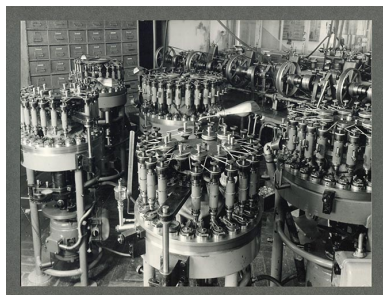
Machines à percer multibroches, années 1960. IVR43_20182500781NUC4A
