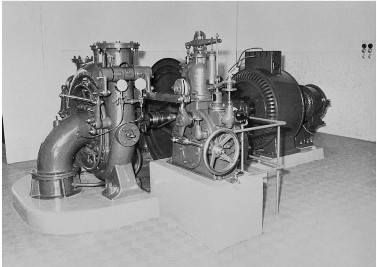
Usine du Flumen. Groupe Escher-Wyss Bréguet de 1911.
