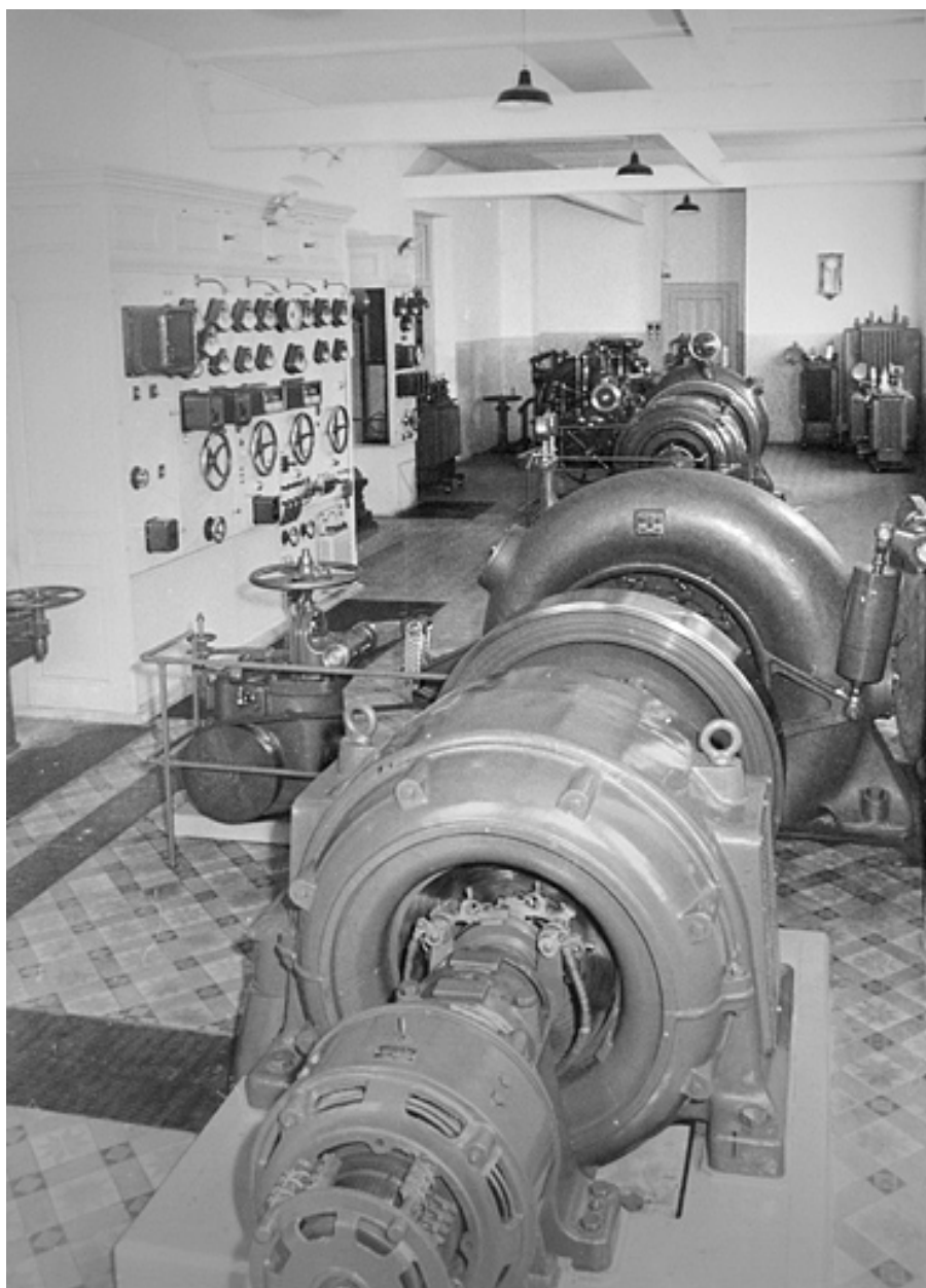
Usine du Flumen. 1940 : la salle des machines (3 groupes).
