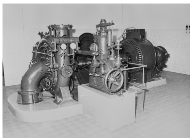
Usine du Flumen. Groupe Escher-Wyss Bréguet de 1911. Phot. Jérôme Mongreville IVR43_19923900014X
