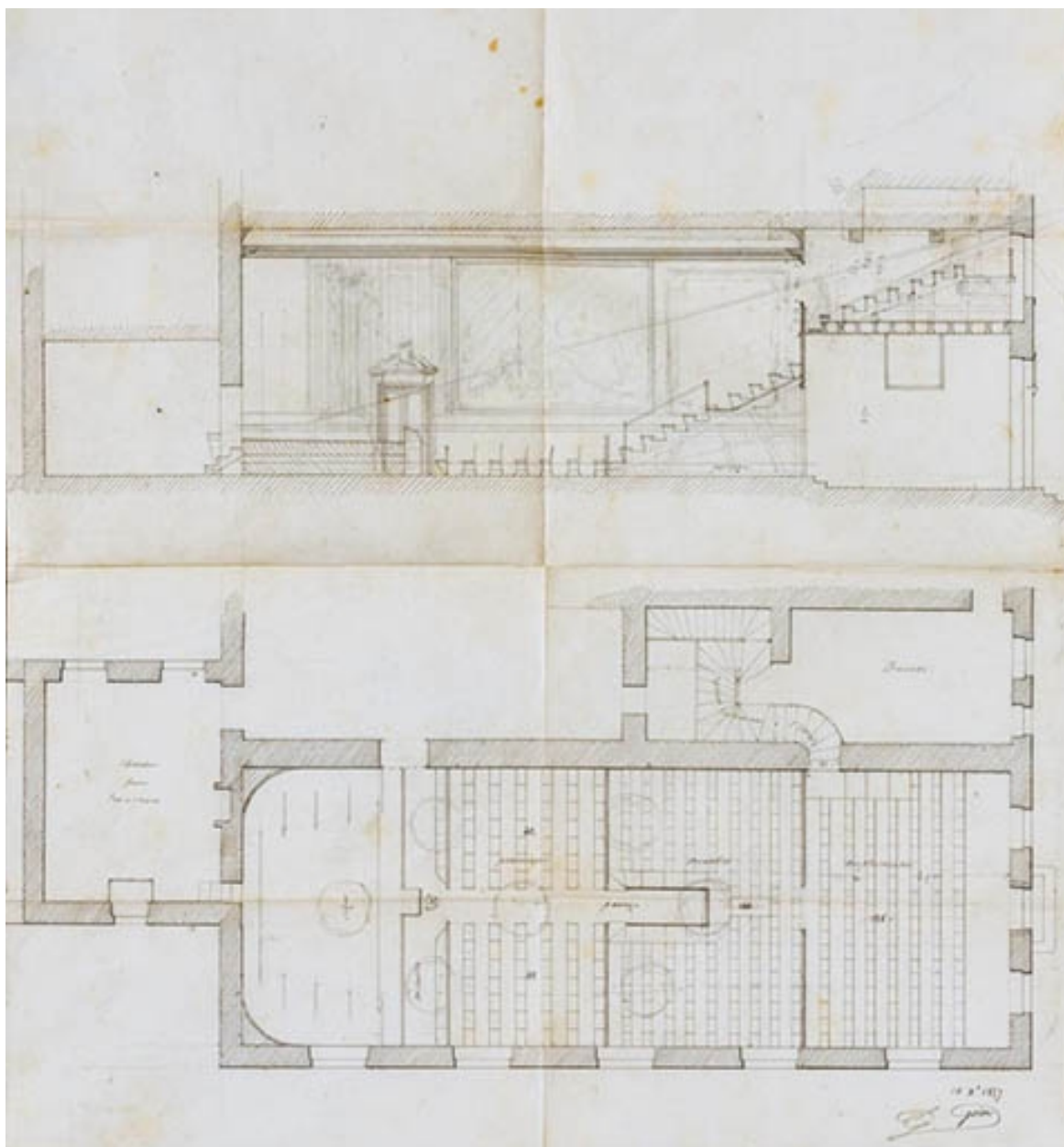
[Plan et coupe de la salle]. 13 décembre 1857.
