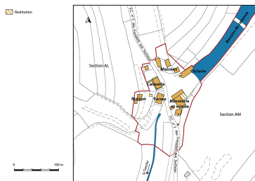
Plan de situation. Extrait du plan cadastral, 2018, sections AL et AM. Dess. Bertrand Turina IVR43_20202500311NUDA
