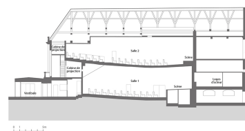
Coupe longitudinale. D'après une coupe non signée non datée fournie par les Services techniques de la Ville. Dess. Aline Thomas IVR26_20238900763NUDA
