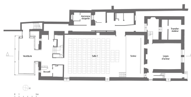
Plan au rez-de-chaussée. D'après un plan non signé non daté fourni par les Services techniques de la Ville. Dess. Aline Thomas IVR26_20238900762NUDA
