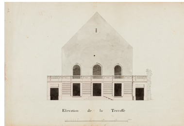
[Projet de salle de réunion et de spectacle dans l'église des capucins]. Elévation de la terrasse. S.d. [entre 1792 et 1795]. Phot. Pierre-Marie Barbe-Richaud, Autr. Jacques Nicolas Caristie IVR26_20238900495NUC4A
