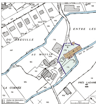
Plan-masse et de situation. Extrait du plan cadastral numérisé, 2005, section A, 1:1250.
