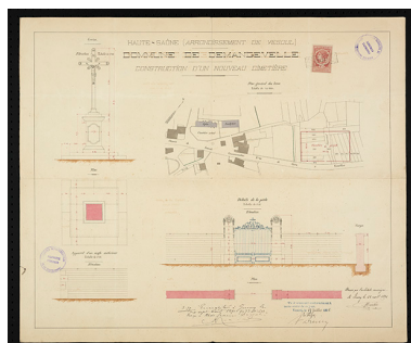
Plan : construction d'un nouveau cimetière. Phot. Sonia Dourlot IVR43_20167000074NUC4A
