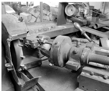
Mandrin gueule de loup et fraise verticale. Phot. Jérôme Mongreville IVR43_20003901056X
