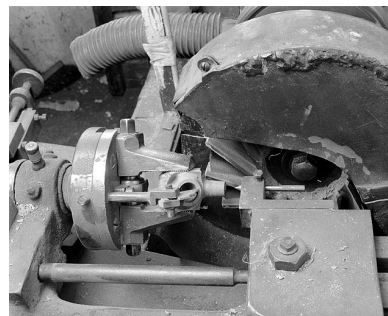
Mandrin gueule de loup et fraise verticale, vue de face en plongée. Phot. Jérôme Mongreville IVR43_20003901054X
