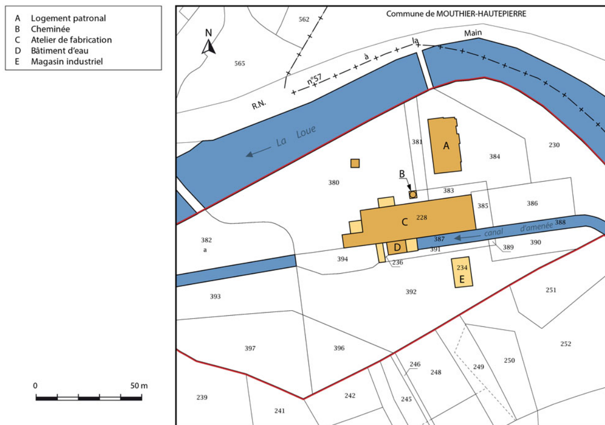
Plan-masse et de situation. Extrait du plan cadastral, 2016, section C.
