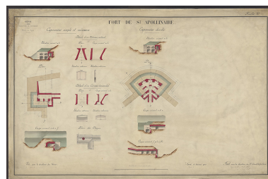
[Fort de Saint Apollinaire : caponnière simple et créneaux et caponnière double]. 1885.
