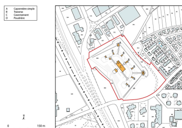
Plan-masse et de situation. Extrait du plan cadastral, 2026, 1/3 000.
