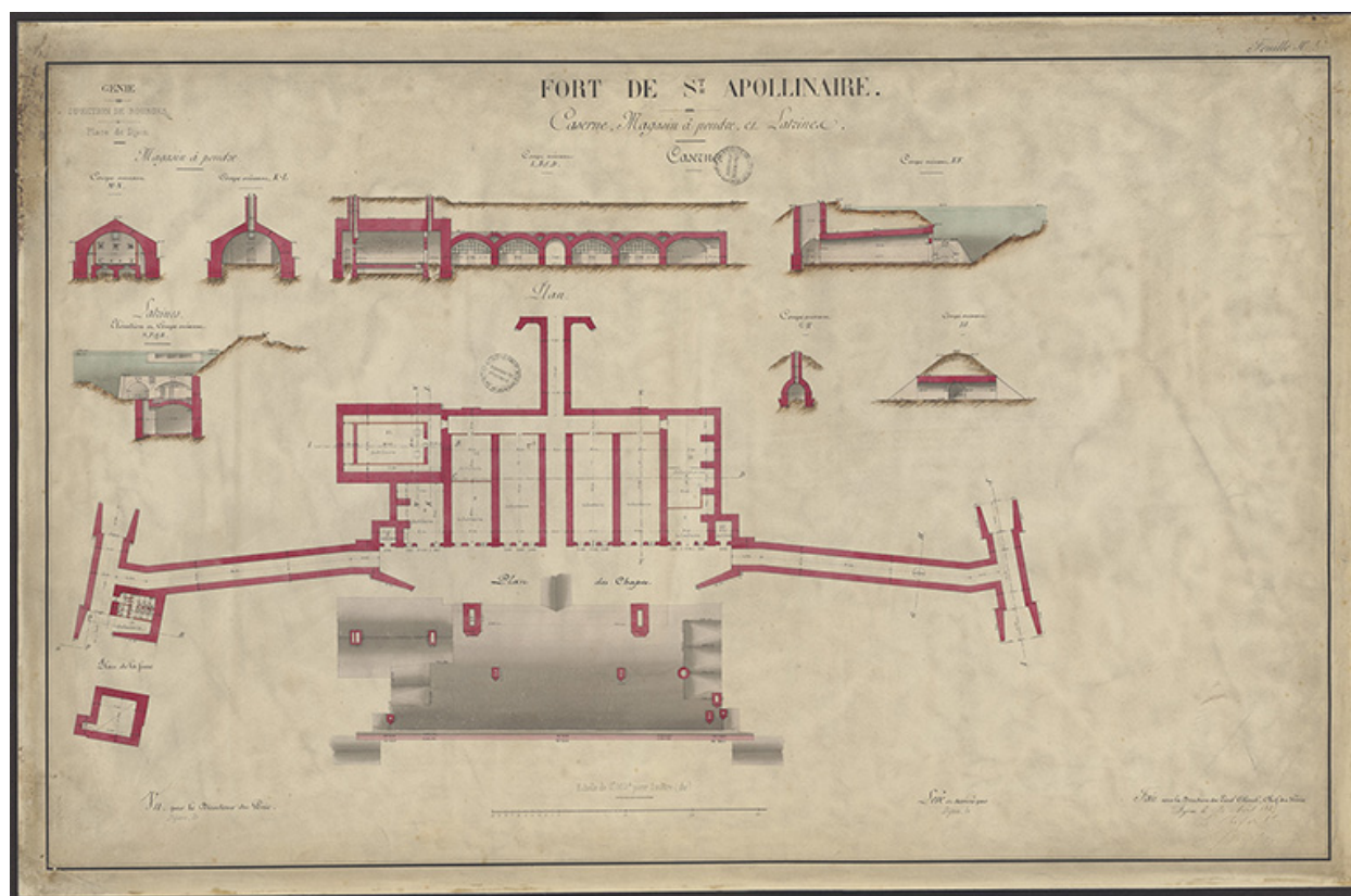
Fort de St Apollinaire. Caserne, magasin à poudre et latrines. 1885.
