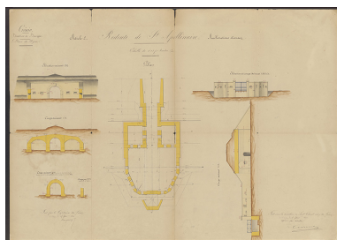
Redoute de St Apollinaire. Améliorations diverses. 1880.
