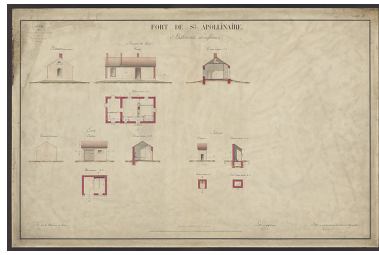
Fort de St Apollinaire. Bâtiments accessoires. S.d. [1898-1905]. Phot. Petot Frédéric, Autr. auteur inconnu IVR26_20252100183NUC4A
