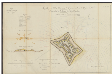
Projets pour 1877 - Travaux de défense autour de Dijon. article 4. Construire la redoute de St Apollinaire. 1877.
