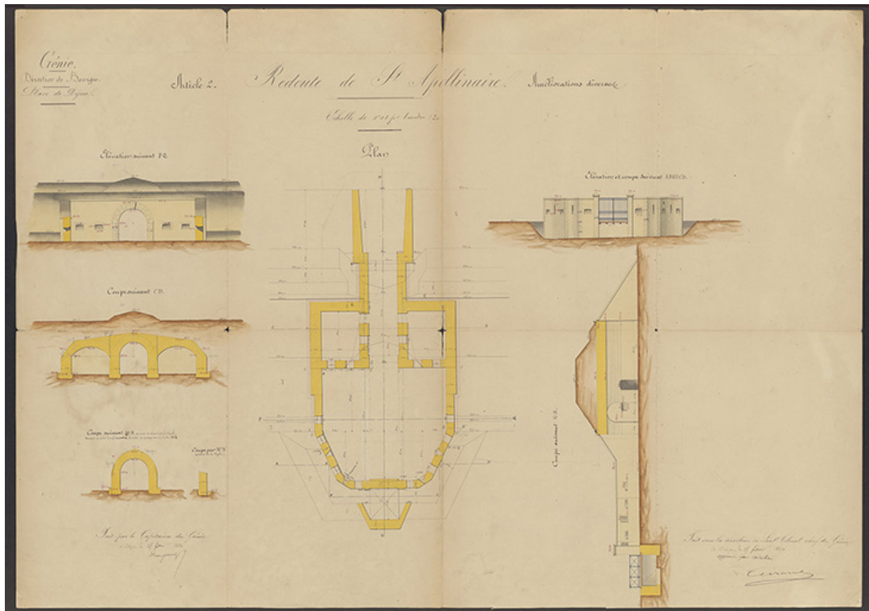
Redoute de St Apollinaire. Améliorations diverses. 1880.
