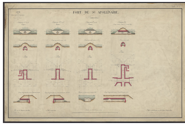
Fort de St Apollinaire. Traverses. 1885. Phot. Petot Frédéric, Autr. auteur inconnu IVR26_20252100186NUC4A
