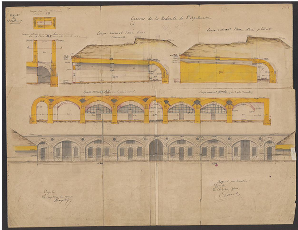
Caserne de la redoute de St Apollinaire. [1877].
