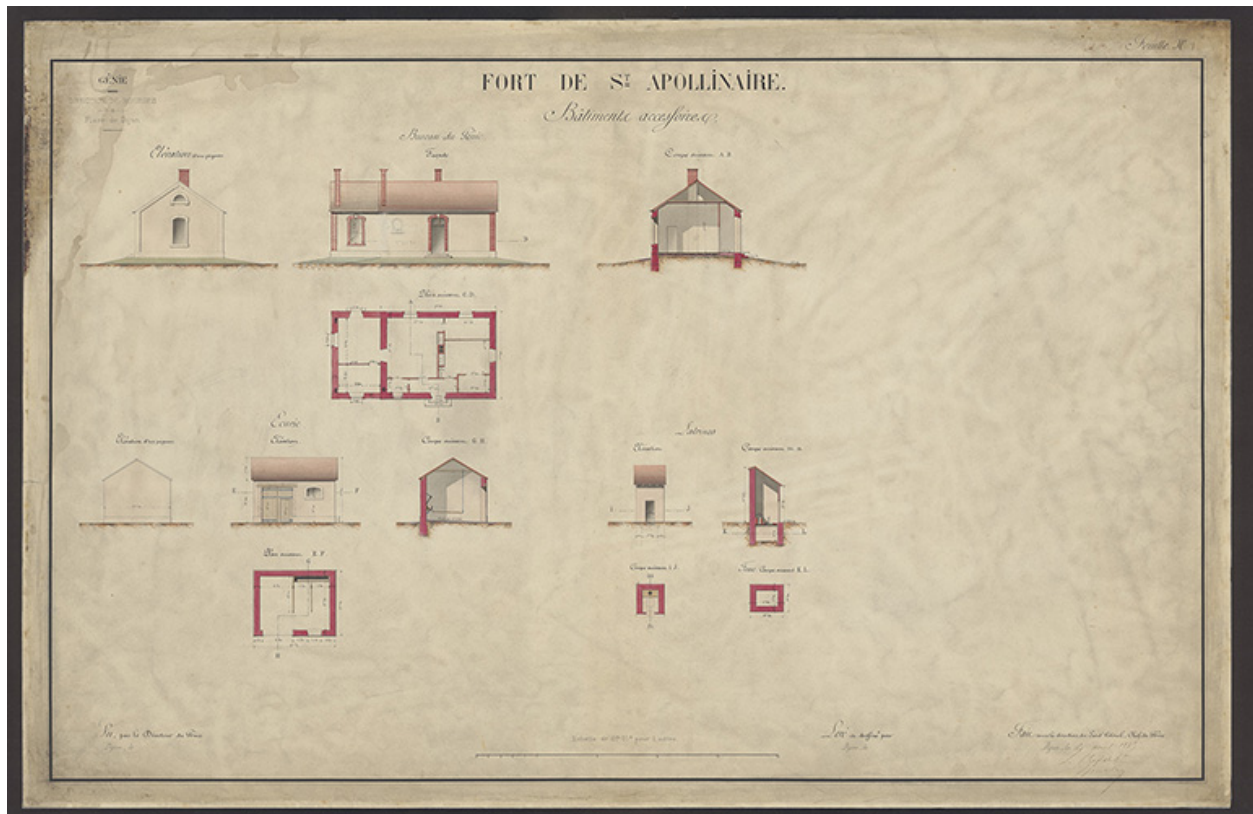
Fort de St Apollinaire. Bâtiments accessoires. S.d. [1898-1905].
