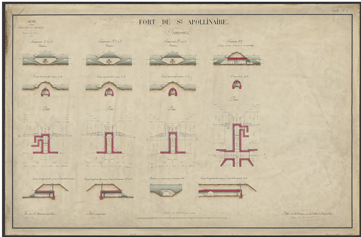
Fort de St Apollinaire. Traverses. 1885.
