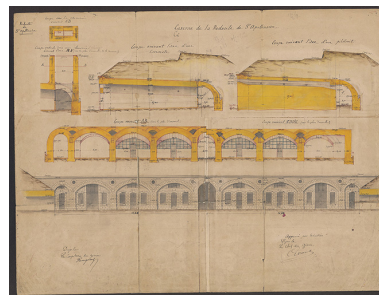
Caserne de la redoute de St Apollinaire. [1877].
