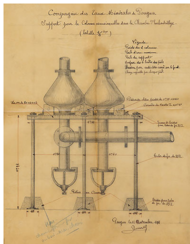
Aménagement de la chambre d'embouteillage (début du 20e siècle). Repro. Pierre-Marie Barbe- Richaud, Autr. Lucas IVR26_20205800189NUC2A
