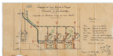
Aménagement de la chambre d'embouteillage (début du 20e siècle). Repro. Pierre-Marie Barbe- Richaud, Autr. Lucas IVR26_20205800190NUC2A
