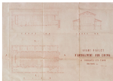
Projet de transformation de l'usine en cinéma (plan et coupes) datant de 1950. Repro. Pierre-Marie Barbe- Richaud, Autr. Robert Riniéri
