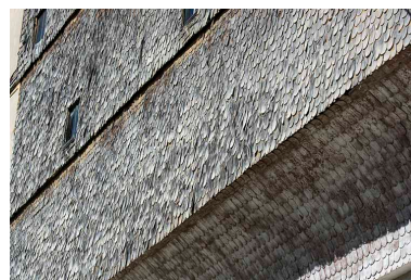
Façade postérieure : rang pendu et essentage de tavaillons. Phot. Sonia Dourlot IVR43_20172500652NUC4A
