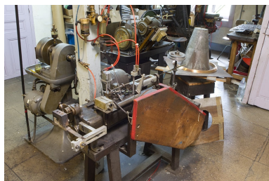
Vue d'ensemble. Le chalumeau était fixé sur le support en aluminium au premier plan. Phot. Yves Sancey IVR43_20103900250NUC2A
