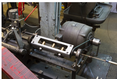
La " toupie " et son moteur. Phot. Yves Sancey IVR43_20103900251NUC2A
