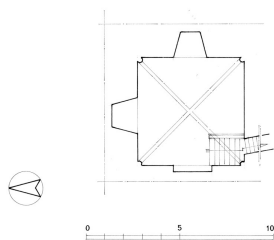
Plan de la crypte. Dess. Alain Morelière IVR26_20128900225A3YY
