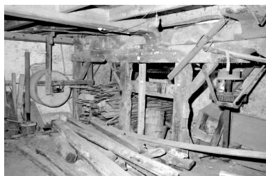
Tonneau de polissage et transmission (2e étage de soubassement). Phot. Laurent Poupard IVR43_19913901267Z
