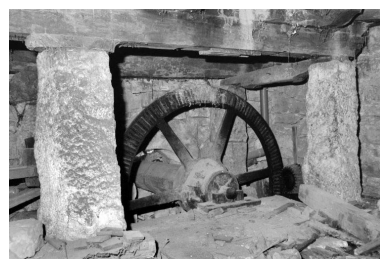
Transmission d'une roue hydraulique (2e étage de soubassement). Phot. Laurent Poupard IVR43_19913901266Z
