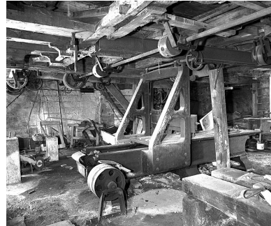
Partie arrière : poulies et engrenages d'entraînement de la table. En côté de l'entretoise, manivelle de réglage en hauteur de la traverse porte-outil. Phot. Yves Sancey IVR43_19943901360X
