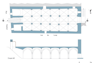
Plan et coupe de la cave. Dess. Mathias Papigny, Dess. Jean-Denis Clabaut IVR43_20132500389NUDA
