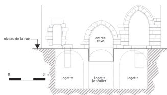
Restitution partielle de l'élévation sur rue. Dess. Mathias Papigny, Dess. Jean-Denis Clabaut IVR43_20132500390NUDA
