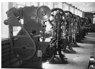
Atelier d'ébauches (section de presses de reprises laiton), vers 1950. IVR43_20182500830NUC4A
