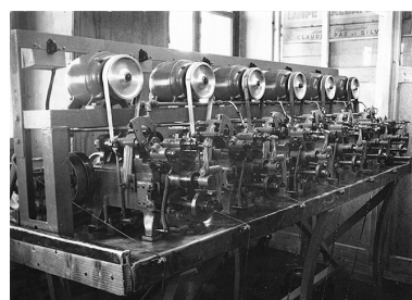
Groupe de décolleteuses automatiques de reprise, vers 1950. IVR43_20182500832NUC4A
