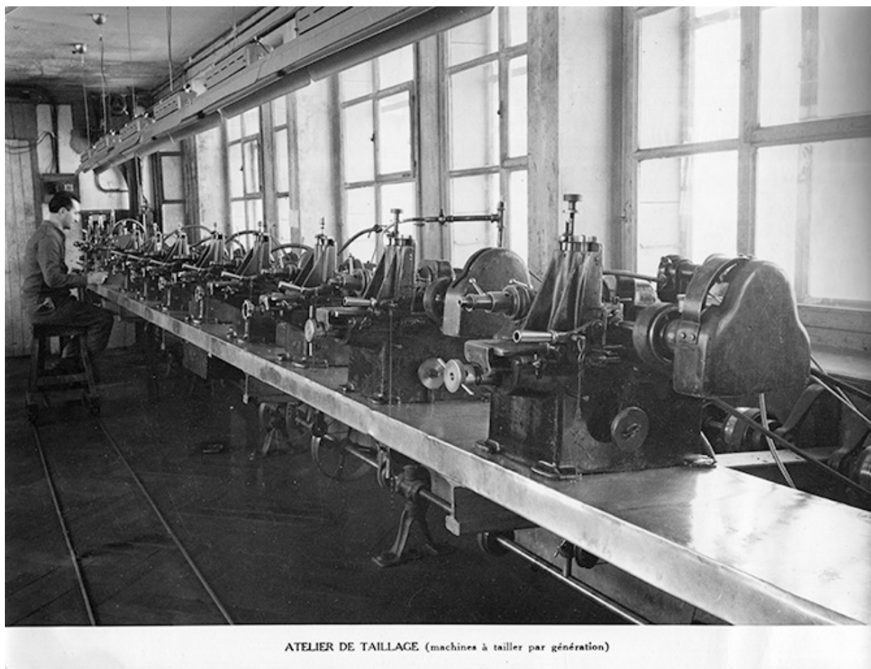
Atelier de taillage (machines à tailler par génération), vers 1950.
