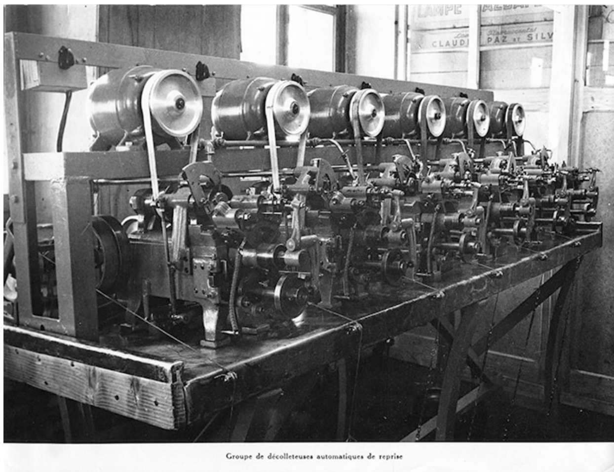
Groupe de décolleteuses automatiques de reprise, vers 1950.
