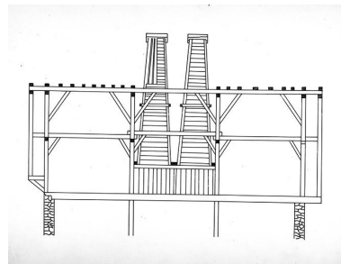
Coupe de la charpente. Phot. Yves Sancey IVR43_19802500039V
