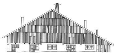
Elévation de la façade postérieure. Phot. Yves Sancey IVR43_19802500038V
