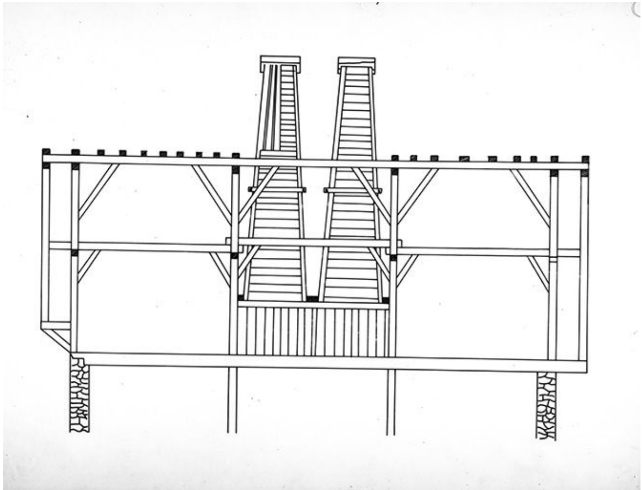
Coupe de la charpente.
