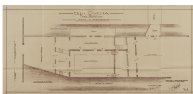
Eden-Cinéma. Plan général. Sorties et dégagements. 1934. Phot. Pierre-Marie Barbe- Richaud, Autr. Roger Charton IVR26_20245800290NUC2A
