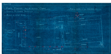
Eden-Cinéma rue St Agnan Cosne. Monsieur Pluviaux propriétaire. Relevé de l'état actuel. Plan du cinéma et des galeries bal. 1922. Phot. Pierre-Marie Barbe- Richaud, Autr. Fernand Boussard IVR26_20245800289NUC2A
