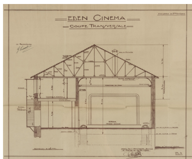
Eden-Cinéma. Coupe transversale. 1934. Phot. Pierre-Marie Barbe- Richaud, Autr. Roger Charton IVR26_20245800291NUC2A
