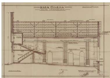
Eden-Cinéma. Coupe longitudinale. 1934. Phot. Pierre-Marie Barbe- Richaud, Autr. Roger Charton IVR26_20245800292NUC4A
