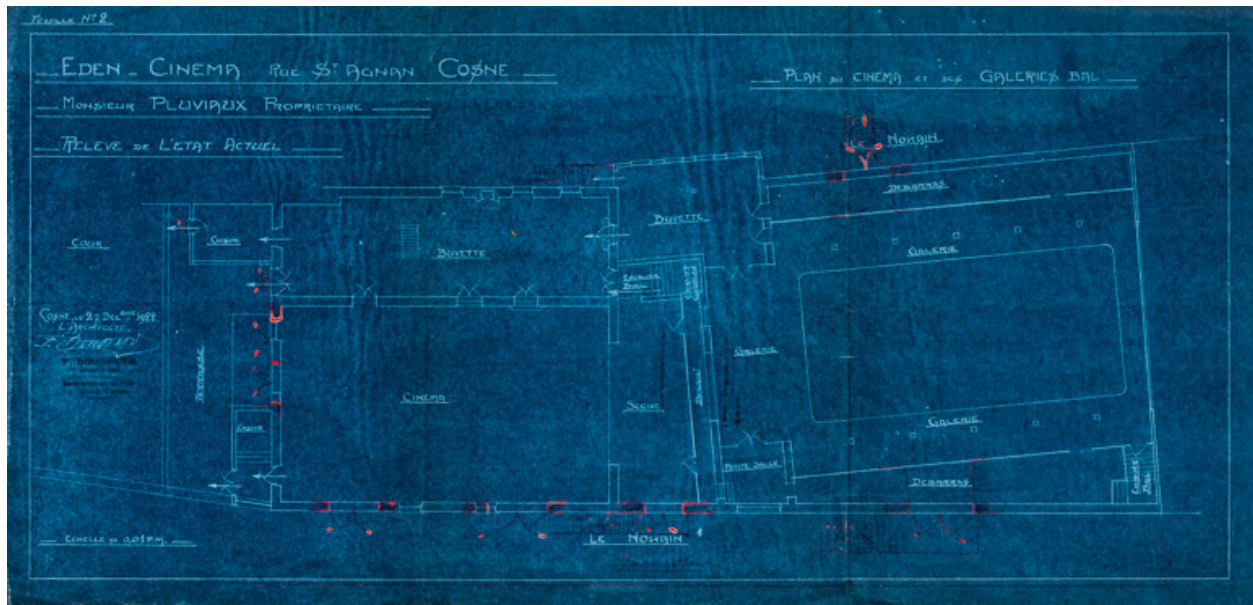
Eden-Cinéma rue St Agnan Cosne. Monsieur Pluviaux propriétaire. Relevé de l'état actuel. Plan du cinéma et des galeries bal. 1922.
