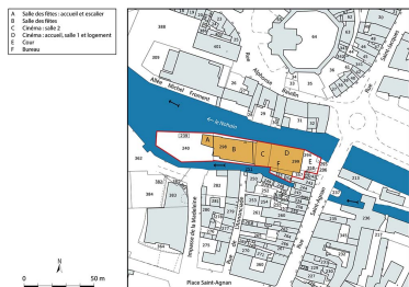
Plan-masse et de situation. Source : Direction générale des Finances Publiques - Cadastre ; mise à jour 2023, section AM, 1/500 agrandi à 1/1 000. Dess. Aline Thomas IVR26_20245800641NUDA
