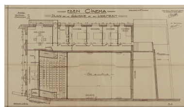
Eden-Cinéma. Plan de la galerie et du logement. 1934. Phot. Pierre-Marie Barbe- Richaud, Autr. Roger Charton IVR26_20245800293NUC4A
