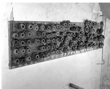
Ratelier de roues dentées pour les cardes, vu de trois quarts. Phot. Yves Sancey IVR43_19943901551X
