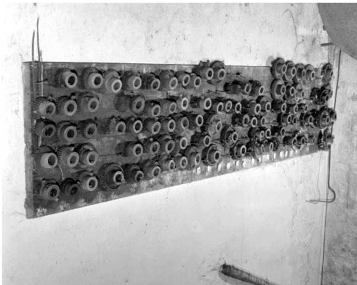
Ratelier de roues dentées pour les cardes, vu de trois quarts.
