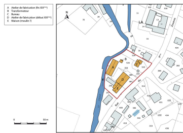
Plan-masse et de situation. Dess. Mathias Papigny IVR43_20132502627NUDA
