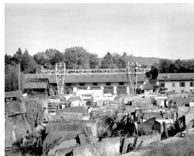
Portique roulant vu de face. Phot. Yves Sancey IVR43_19933900320X
