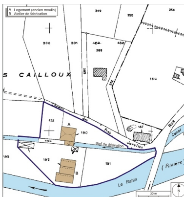
Plan-masse et de situation. Extrait du plan cadastral numérisé, 2008, section AK, échelle 1:1000. Source : Direction générale des Finances Publiques - Cadastre ; mise à jour : 2008. Dess. André Céréza IVR43_20087000171NUDA
