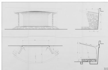
[Plan, coupes et élévation]. S.d. [1969]. Phot. Pierre-Marie Barbe- Richaud, Autr. Guy Devertu IVR26_20238900060NUC4A
