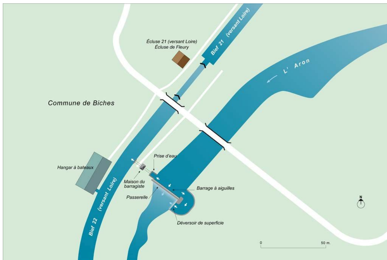
Carte schématique du barrage de Fleury.
