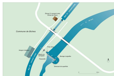
Carte schématique du barrage de Fleury. Dess. Alain Morelière IVR26_20145800021NUDA
