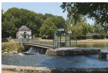
Vue d'ensemble du barrage. Au premier plan, le déversoir et au fond, la maison du barragiste. Phot. Thierry Kuntz IVR26_20135800229NUC4A
