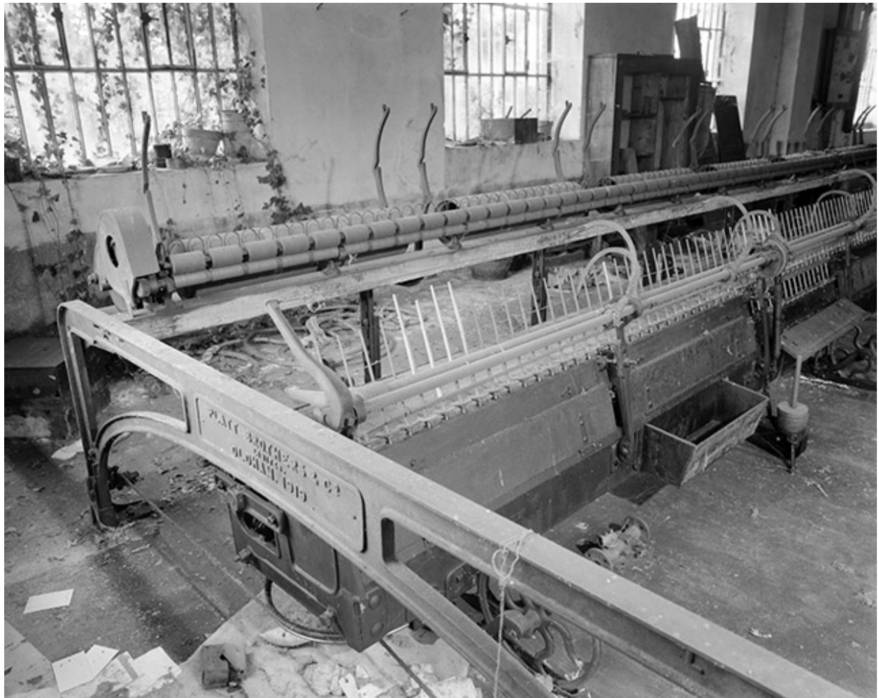
Extrémité du chariot du module de gauche.
