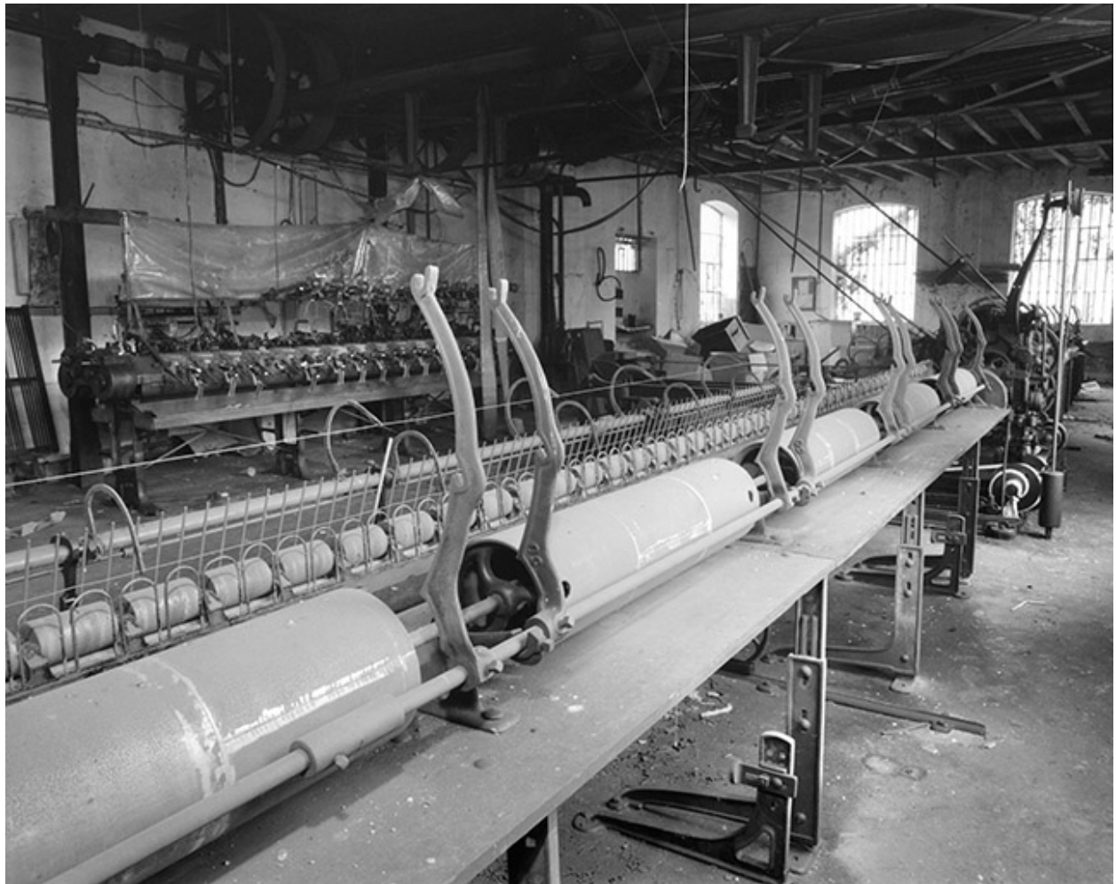
Ratelier du module de droite. Au premier plan, tambours (horizontaux) et supports des cannelles (verticaux).
