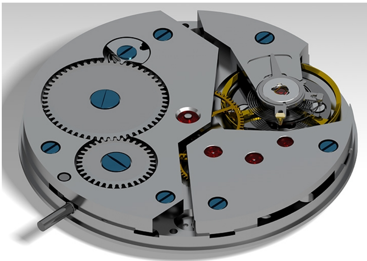
Montre de gousset mécanique : mouvement côté fond.
