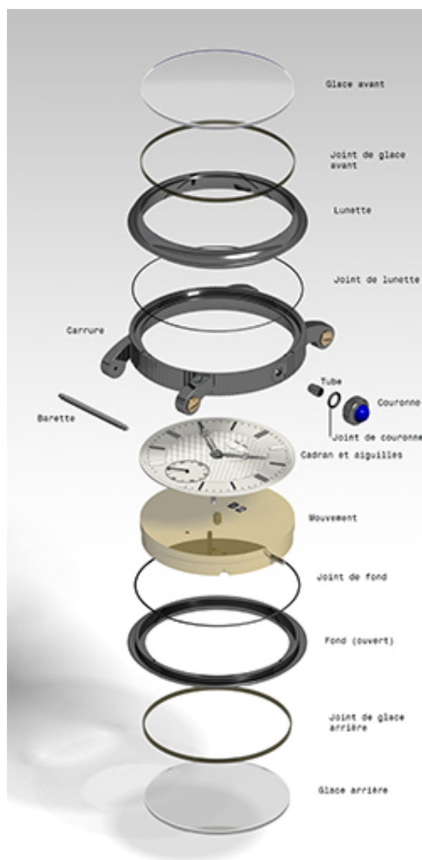
Montre-bracelet : présentation éclatée de l'habillage.
