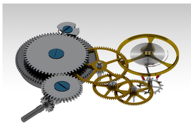
Chaîne cinématique d'une montre mécanique (sans ombrage). Dess. William Berthet IVR43_20202500246NUC4A
