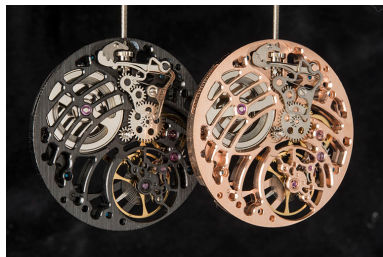
Deux mouvements squelette (Unitas 6498 avec squelettage Arte). Phot. Sonia Dourlot IVR43_20182501160NUC4A
