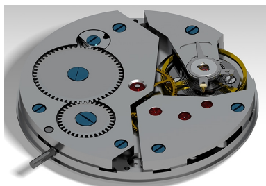
Montre de gousset mécanique : mouvement côté fond. Dess. William Berthet IVR43_20202500256NUC4A
