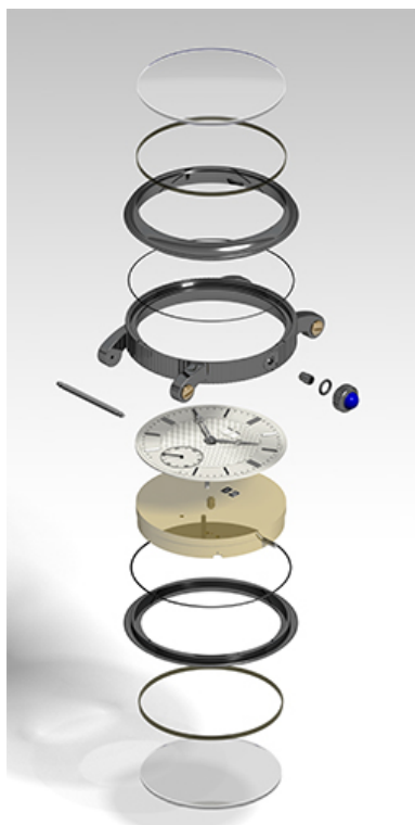
Montre-bracelet : présentation éclatée de l'habillage (sans identification des pièces).
