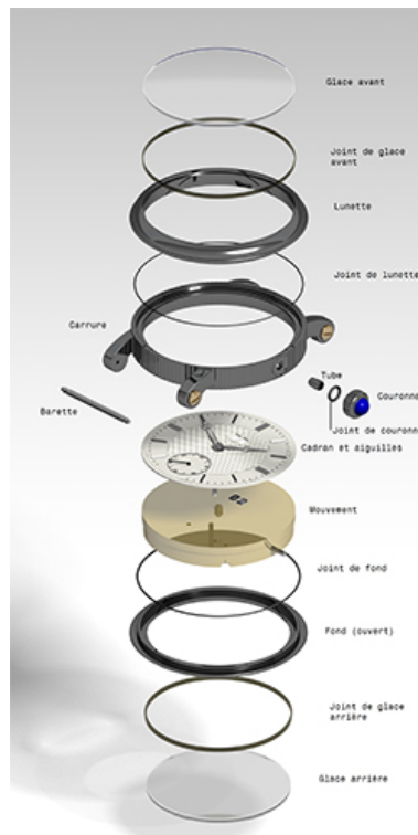
Montre-bracelet : présentation éclatée de l'habillage. Dess. William Berthet
