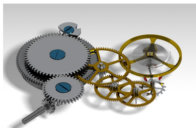
Chaîne cinématique d'une montre mécanique. Dess. William Berthet IVR43_20202500245NUC4A
