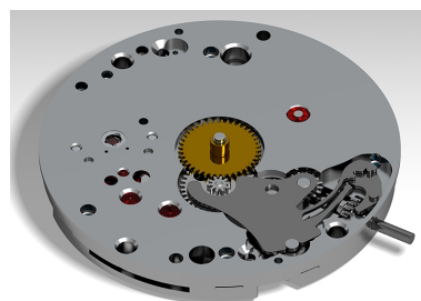
Montre de gousset mécanique : mouvement côté cadran. Dess. William Berthet IVR43_20202500257NUC4A
