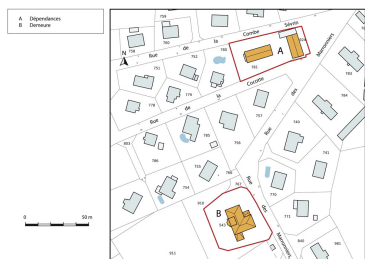
Plan-masse et de situation. Dess. Mathias Papigny IVR43_20132502551NUDA
