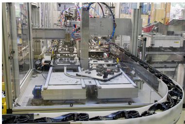
Site récent : machine de l'atelier d'injection zamak. Phot. Yves Sancey IVR43_20132502475NUC2A
