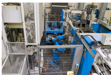
Site ancien : machine de l'atelier d'injection zamak. Phot. Yves Sancey IVR43_20132502458NUC2A
