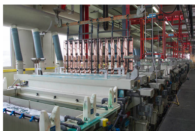
Site ancien : chaîne de chromage. Phot. Yves Sancey IVR43_20132502460NUC2A
