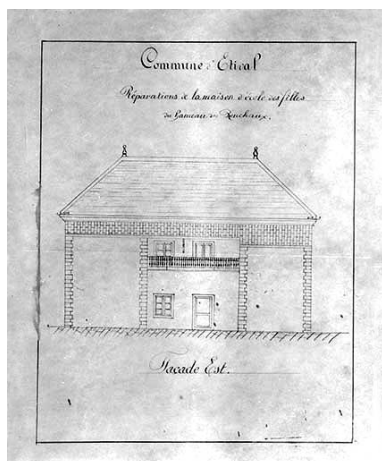
Commune d'Etival. Réparations à la maison d'Ecole des Filles [...] Façade est. Phot. Jérôme Mongreville, Phot. Comoy IVR43_19963900196X
