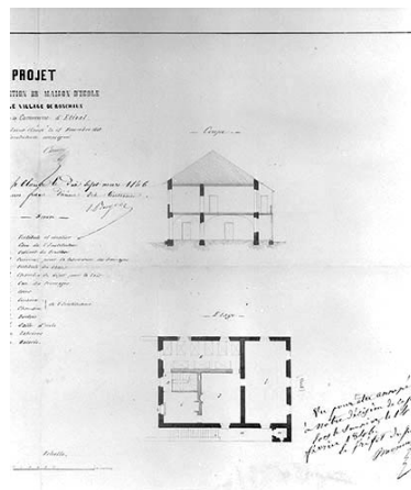
Projet d'appropriation de Maison d'Ecole [...] [plan à l'étage et coupe]. Phot. Jérôme Mongreville, Phot. Comoy IVR43_19963900192X
