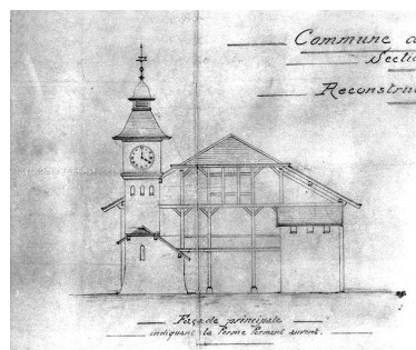
Commune d'Etival [...] [détail : élévation de la façade est]. Reconstruction de la toiture du chalet incendié [détail : élévation de la façade est]. Phot. Jérôme Mongreville, Phot. Jules Pelletier IVR43_19963900195X
