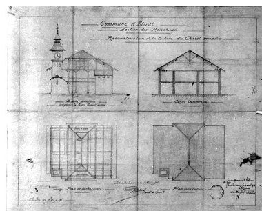
Commune d'Etival [...] [plans, coupe et élévation]. Reconstruction de la toiture du chalet incendié [plans, coupe et élévation]. Phot. Jérôme Mongreville, Phot. Jules Pelletier IVR43_19963900194X
