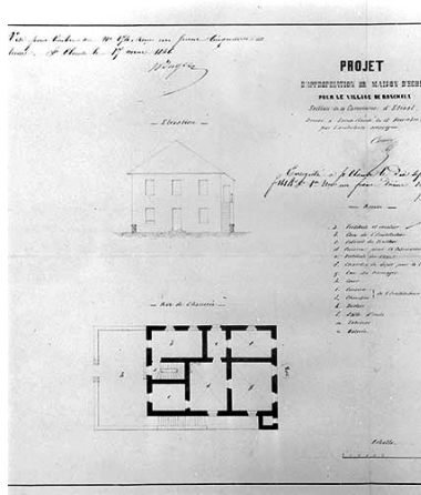
Projet d'appropriation de Maison d'Ecole [...] [plan au rez-de-chaussée et élévation]. Phot. Jérôme Mongreville, Phot. Comoy IVR43_19963900191X
