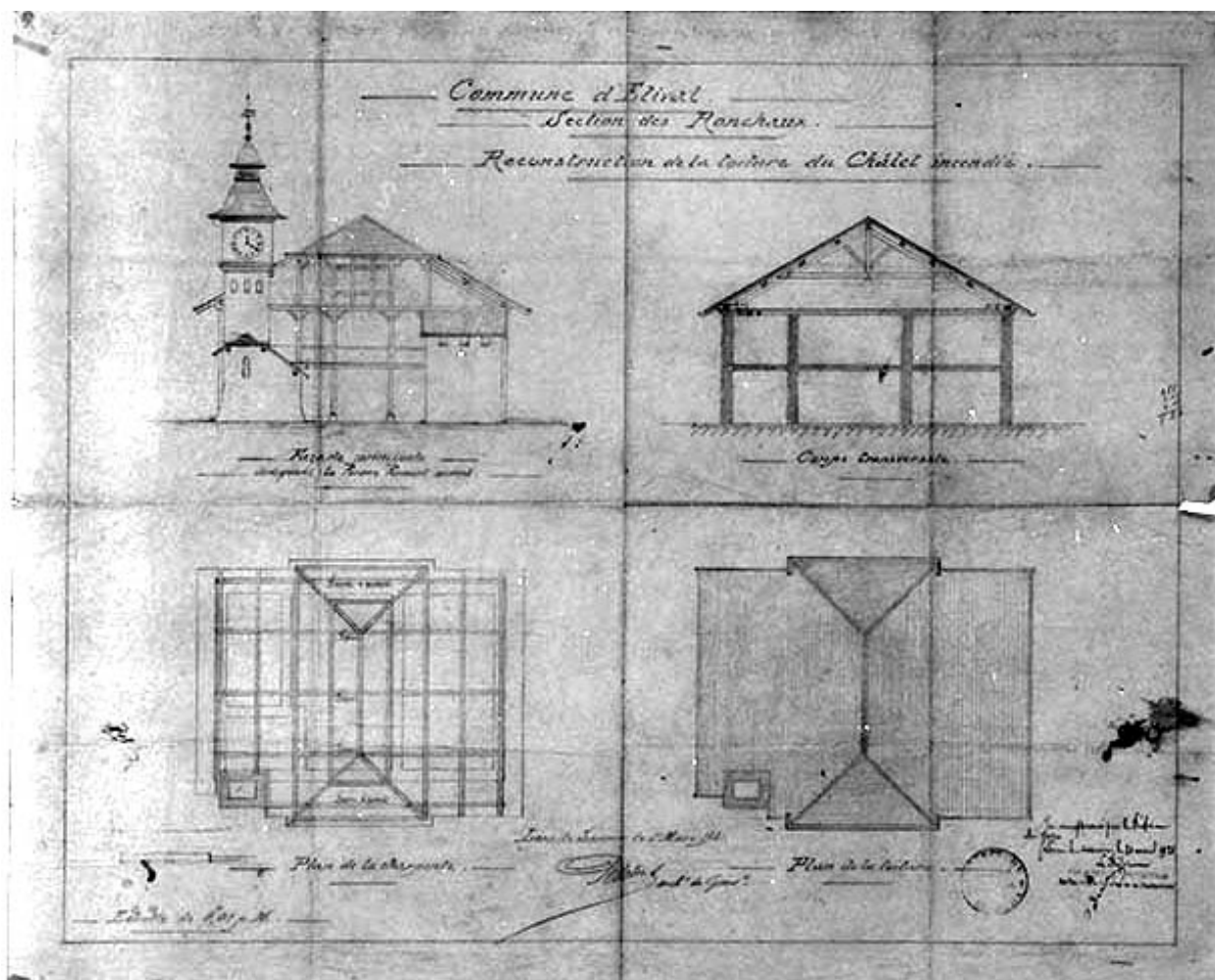
Commune d'Etival [...] Reconstruction de la toiture du chalet incendié [plans, coupe et élévation].
