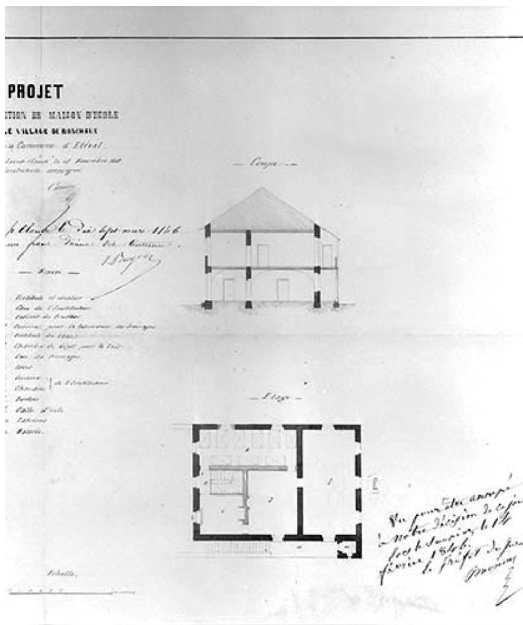
Projet d'appropriation de Maison d'Ecole [...] [plan à l'étage et coupe].
