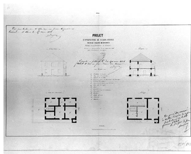
Projet d'appropriation de Maison d'Ecole [...] [plans, coupe et élévation]. Phot. Jérôme Mongreville, Autr. NEPASUTILISERComoy (architecte) IVR43_19963900190X
