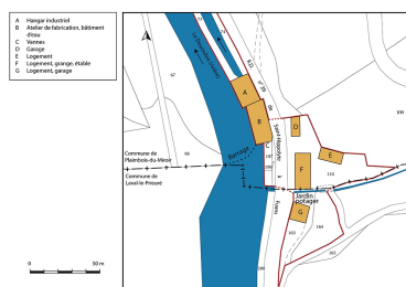
Plan-masse et de situation. Extrait du plan cadastral, Plaimbois-du-Miroir, 2018, section B et Laval-le-Prieuré, 2019, section B. Dess. Bertrand Turina IVR43_20202500329NUDA
