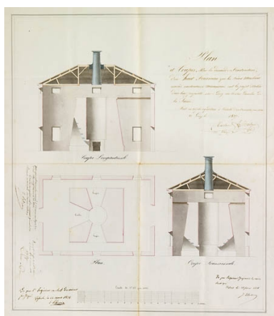
Plan et coupes pour la demande en construction d'un haut fourneau que les frères Marland associés, constructeurs mécaniciens, ont le projet d'établir dans leur propriété, sise à Gray, sur la rive gauche de la Saône. Phot. Jérôme Mongreville IVR43_20097000067NUC2A
