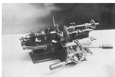
[Machine à rectifier les siettes ?], 2e quart 20e siècle ? (après 1936). Phot. Yves Sancey, Autr. Henri Patois IVR43_20132501953NUC2A
