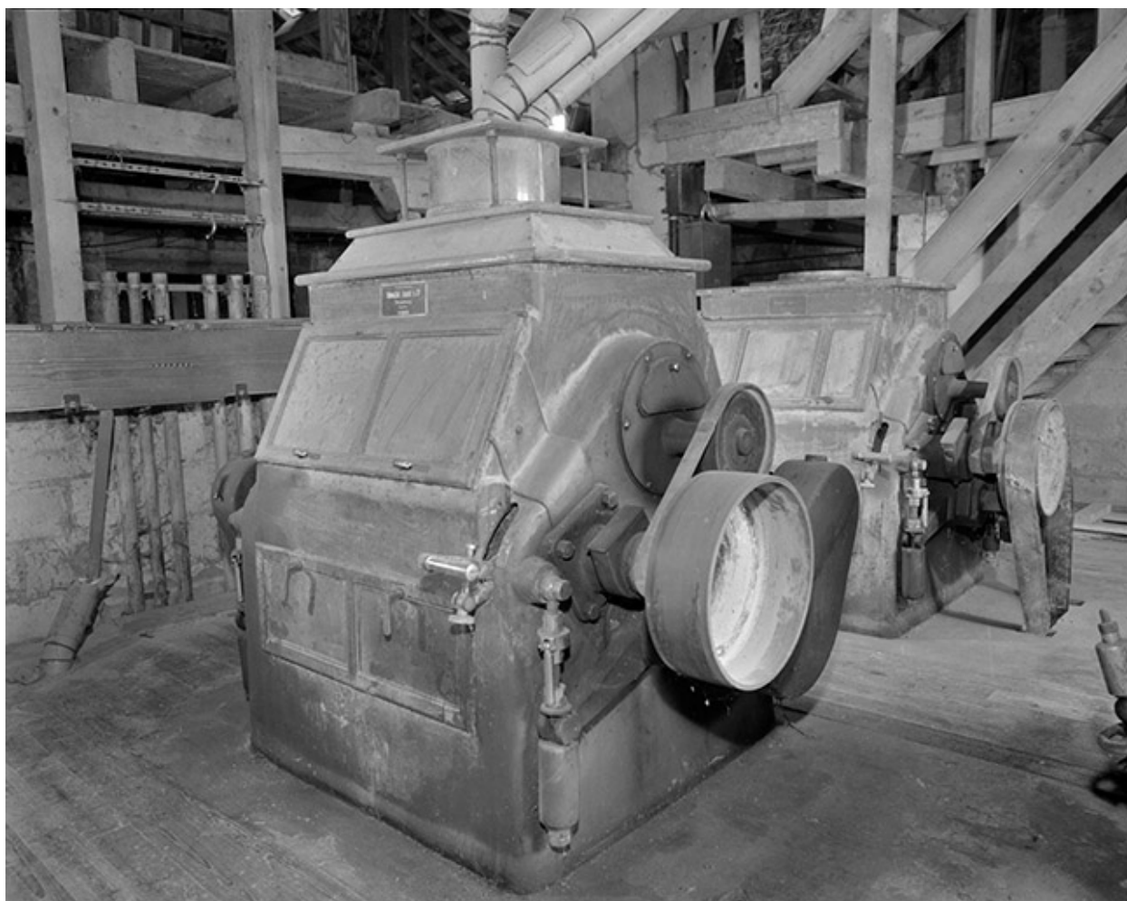
Appareil à cylindres Schneider, Jacquet et Cie (Strasbourg).
