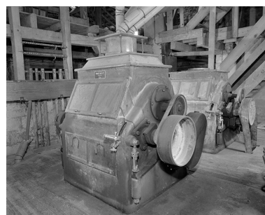
Appareil à cylindres Schneider, Jacquet et Cie (Strasbourg). Phot. Jérôme Mongreville IVR43_19963900068X
