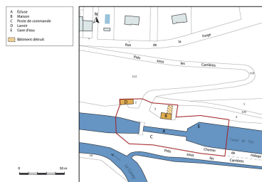
Plan masse et de situation. Dess. Mathias Papigny IVR43_20167000166NUDA
