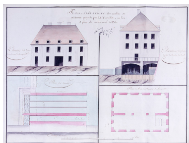
Plans et élévations des moulins et bâtiments projetés par M. Vermillet, au lieu et place du Moulin-Neuf à Dôle. Phot. Yves Sancey IVR43_19903901008XA
