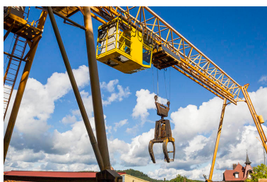
Portique roulant : cabine de commande et pince. Phot. Yves Sancey IVR43_20132501735NUC2A
