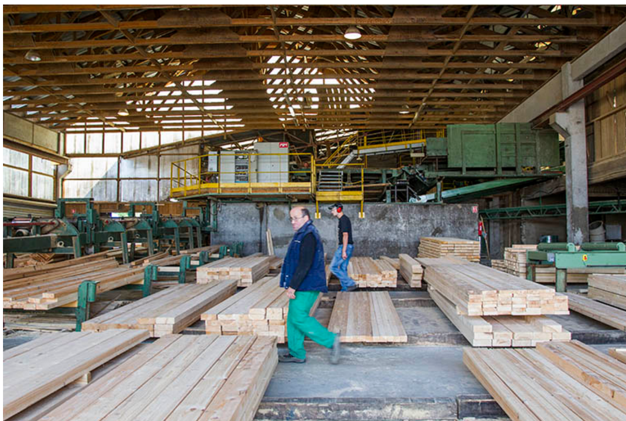
Atelier de triage et d'empilage (E) : intérieur. Au fond en hauteur, l'installation de sciage.
