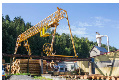
Le portique roulant sur son chemin de roulement. A droite l'atelier de débitage (M). Phot. Yves Sancey IVR43_20132501727NUC2A
