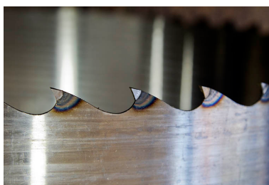
Atelier d'affûtage (K) : détail d'une lame de scie à ruban à double denture.
