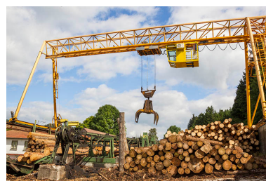
Portique roulant : déplacement de la pince. Phot. Yves Sancey IVR43_20132501721NUC2A
