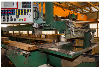
Atelier de triage et d'empilage (E) : scie circulaire de l'installation de sciage. Phot. Yves Sancey IVR43_20132501740NUC2A
