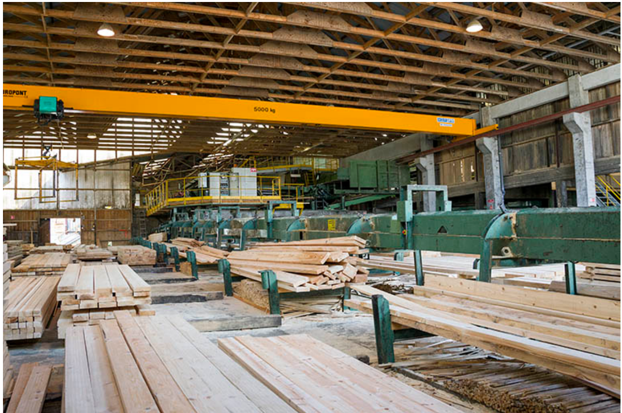
Atelier de triage et d'empilage (E) : intérieur.
