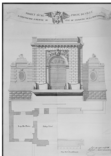
Projet non réalisé de N. Lenoir Le Romain : plan et élévation côté faubourg. Phot. Jean-Luc Duthu, Autr. N. Lenoir Le Romain IVR26_19882101564V
