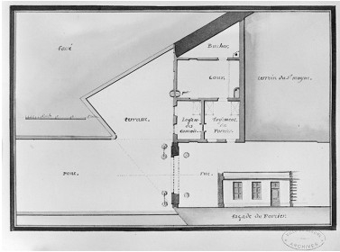
Plan et élévation de la maison du portier par D. Quinard, projet du 18 avril 1782. Phot. Jean-Luc Duthu, Autr. D. Quinard IVR26_19882101556X
