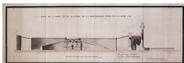
Projet non réalisé de N. Lenoir Le Romain : coupe de la porte. 1764. Phot. Jean-Luc Duthu, Autr. N. Lenoir Le Romain IVR26_19882101559ZA
