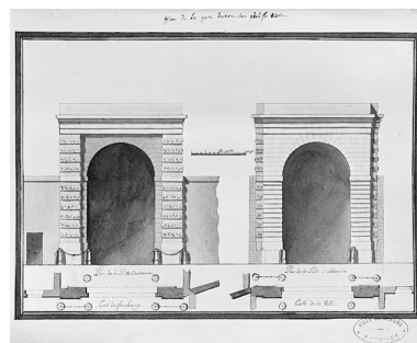
Elévation de la porte par D. Quinard, projet du 18 avril 1782. Phot. Jean-Luc Duthu, Autr. D. Quinard
