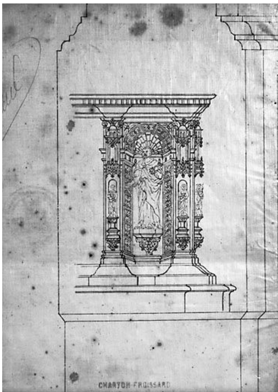
Maître-autel : socle de saint Pierre. Dessin, par Charton-Froissard, 1879.
