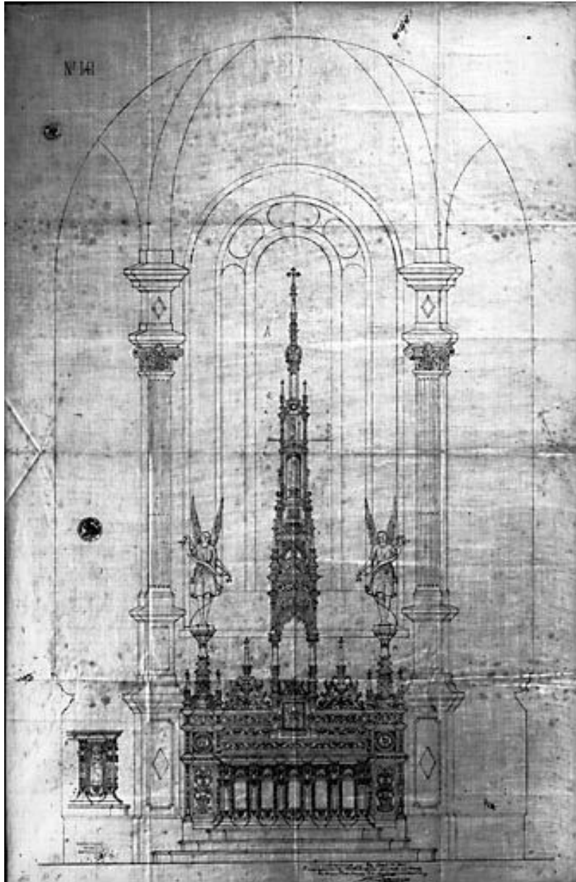
Elévation du maître-autel. Dessin, par Charton-Froissard, 1879
