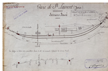
Gare de St Laurent (Jura). Serrures Bouré [plan], 1938. Phot. Yves Sancey IVR43_20073900348NUCA
