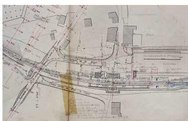
Plan général de la gare de St Laurent [détail de la partie gauche], décennie 1880. Phot. Yves Sancey IVR43_20073900346NUCA
