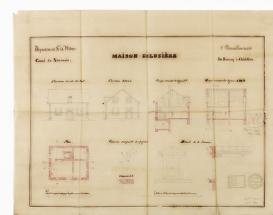
"Maison éclésièr de Bernay à Châtillon". Plan, coupe et élévation et détail de la lucarne. (Archives VNF-direction territoriale Centre-Bourgogne ; subdivision de Corbigny)
