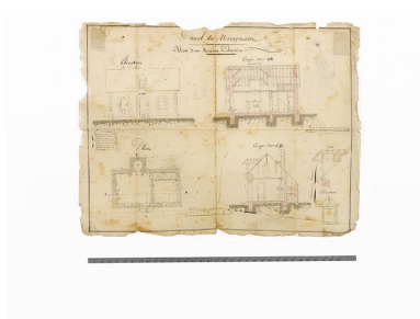
"Plan d'une maison éclusière double". Plan, coupe et élévation (sur laquelle il est précisé "n°30"). (Archives VNF-direction territoriale Centre- Bourgogne ; subdivision de Corbigny)
