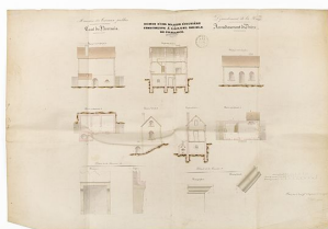
"Dessin d'une maison éclésièr construite à l'écluse double de Chavance". Plan, coupe et élévation (avec détails de la cheminée et de la corniche). (Archives VNF-direction territoriale Centre-Bourgogne ; subdivision de Corbigny)
