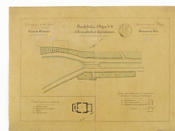
"Plan de l'écluse d'Orgue n°11 et de ses abords et dépendances". Plan général du site d'écluse et détail de la maison éclésièr. (Archives VNF-direction territoriale Centre-Bourgogne ; subdivision de Corbigny)
