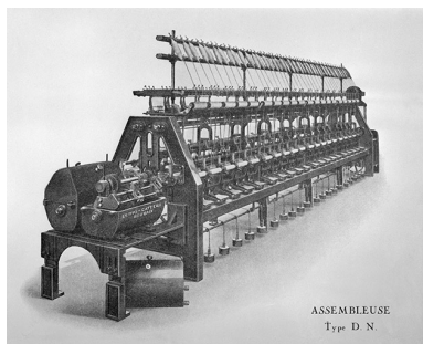
Assembleuse type D.N. Phot. Yves Sancey IVR43_19953900119X
