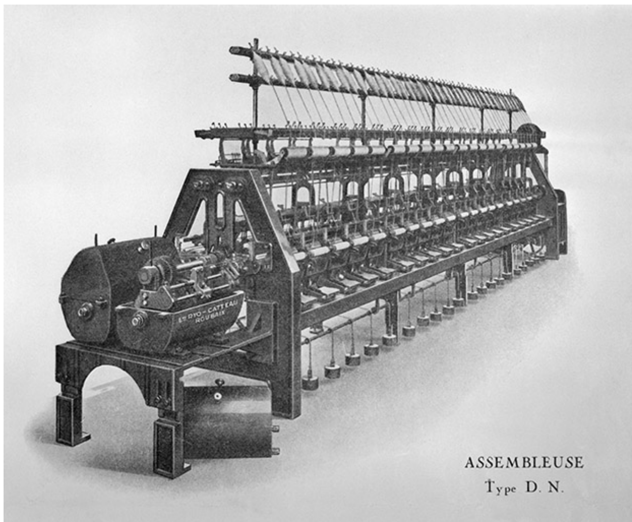
Assembleuse type D.N.
