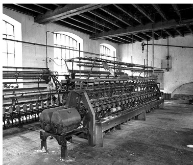
Vue d'ensemble. Phot. Yves Sancey IVR43_19943901490X
