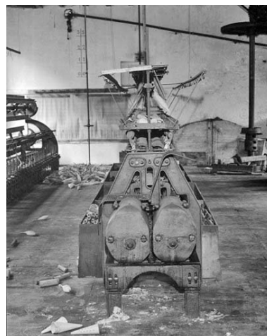
Extrémité de la machine. Phot. Yves Sancey IVR43_19943901491X
