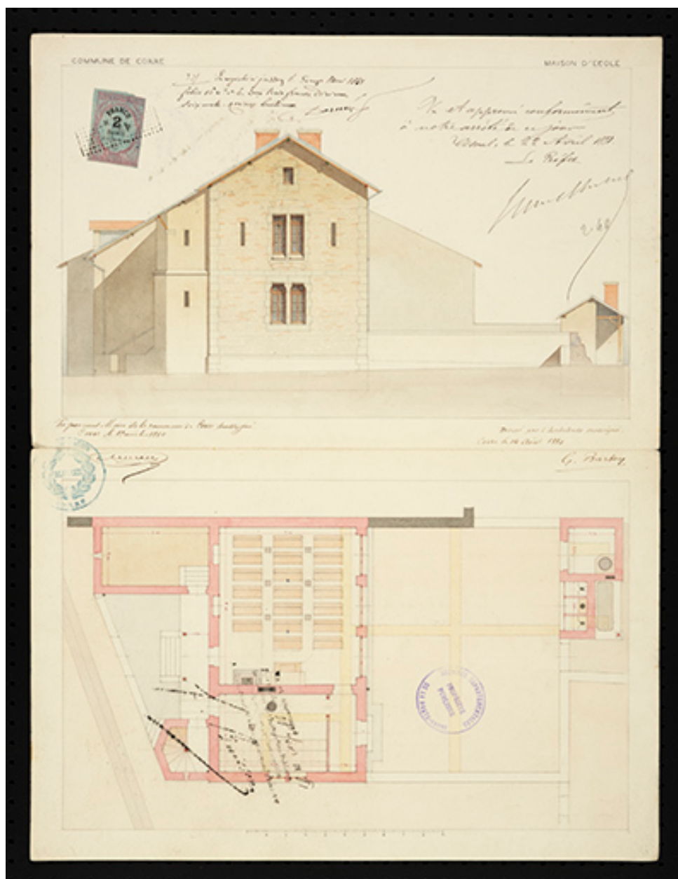
Plans des l'école de filles établis par G. Barbey en 1880 : élévation des pignons et côté ouest, plan du rez-de-chaussée.
