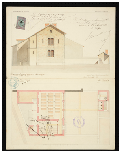
Plans des l'école de filles établis par G. Barbey en 1880 : élévation des pignons et côté ouest, plan du rez-de-chaussée. Phot. Sonia Dourlot IVR43_20167000094NUC4A
