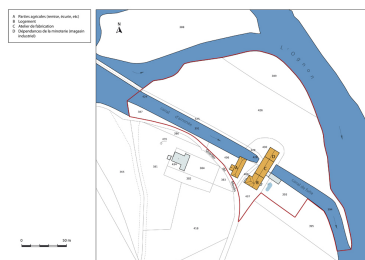
Plan-masse et de situation, extrait du plan cadastral, 2014, section B. Dess. Mathias Papigny IVR43_20142501924NUDA
