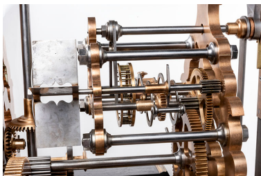
Mouvement : détail du mécanisme.
