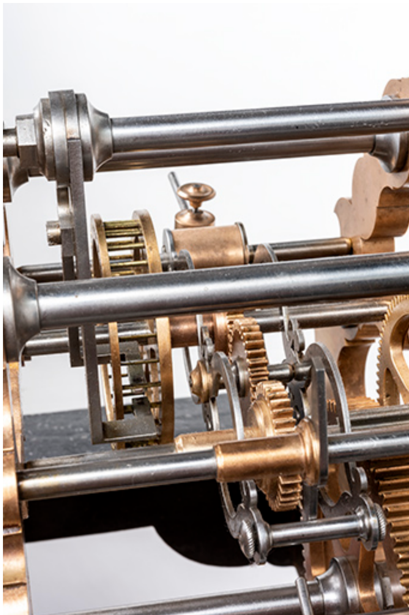
Mouvement : détail de l'échappement.
