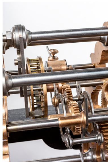
Mouvement : détail de l'échappement.
